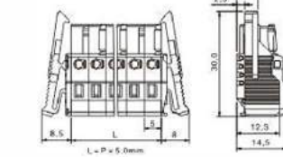
2-24通道孔型连接器带卡接钩 (防错) KF450A
