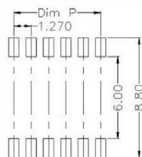
P. C. B. LAYOUT
