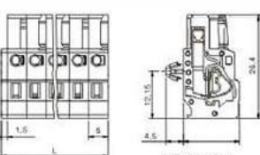
2-24通道孔型连接器带卡接钩 (防错) KF450A
