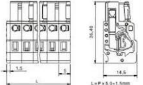
2-24通道孔型连接器带固定器 (防错) KF450B
