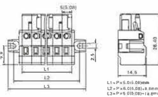
2-24通道孔型连接器带固定器 KF450B1/KF458B1
