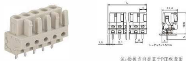
2-24通道孔型插头带直型焊针 (防错)
