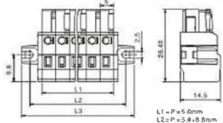
2-24通道孔型连接器带固定器 (防错) KF450B
